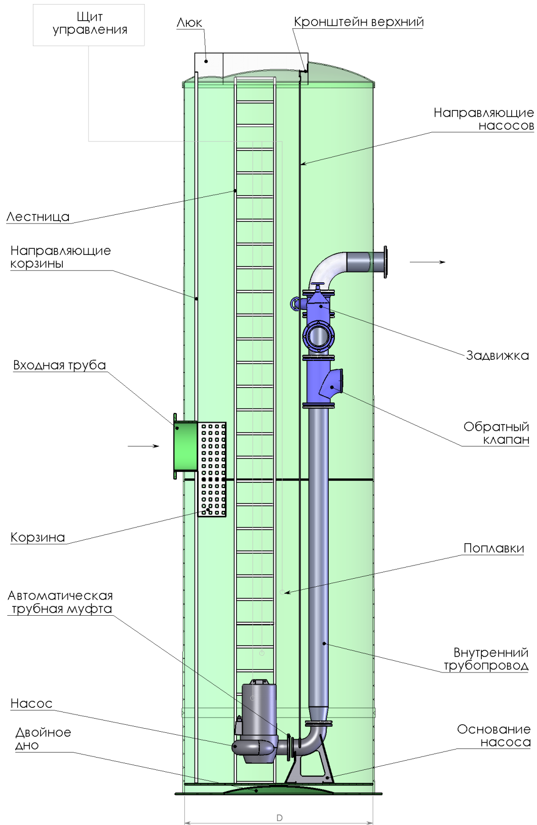
Рис.1 Канализационной насосной станции.
