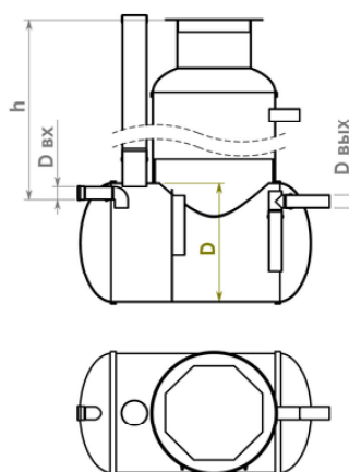
Горизонтальный жиросепаратор
