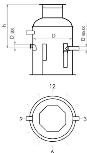
Вертикальный жиросепаратор
