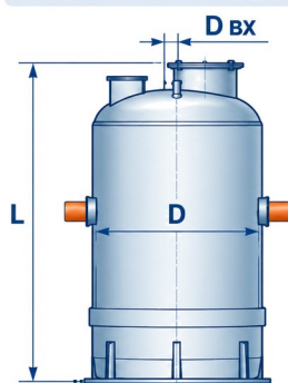
Вертикальная установка
